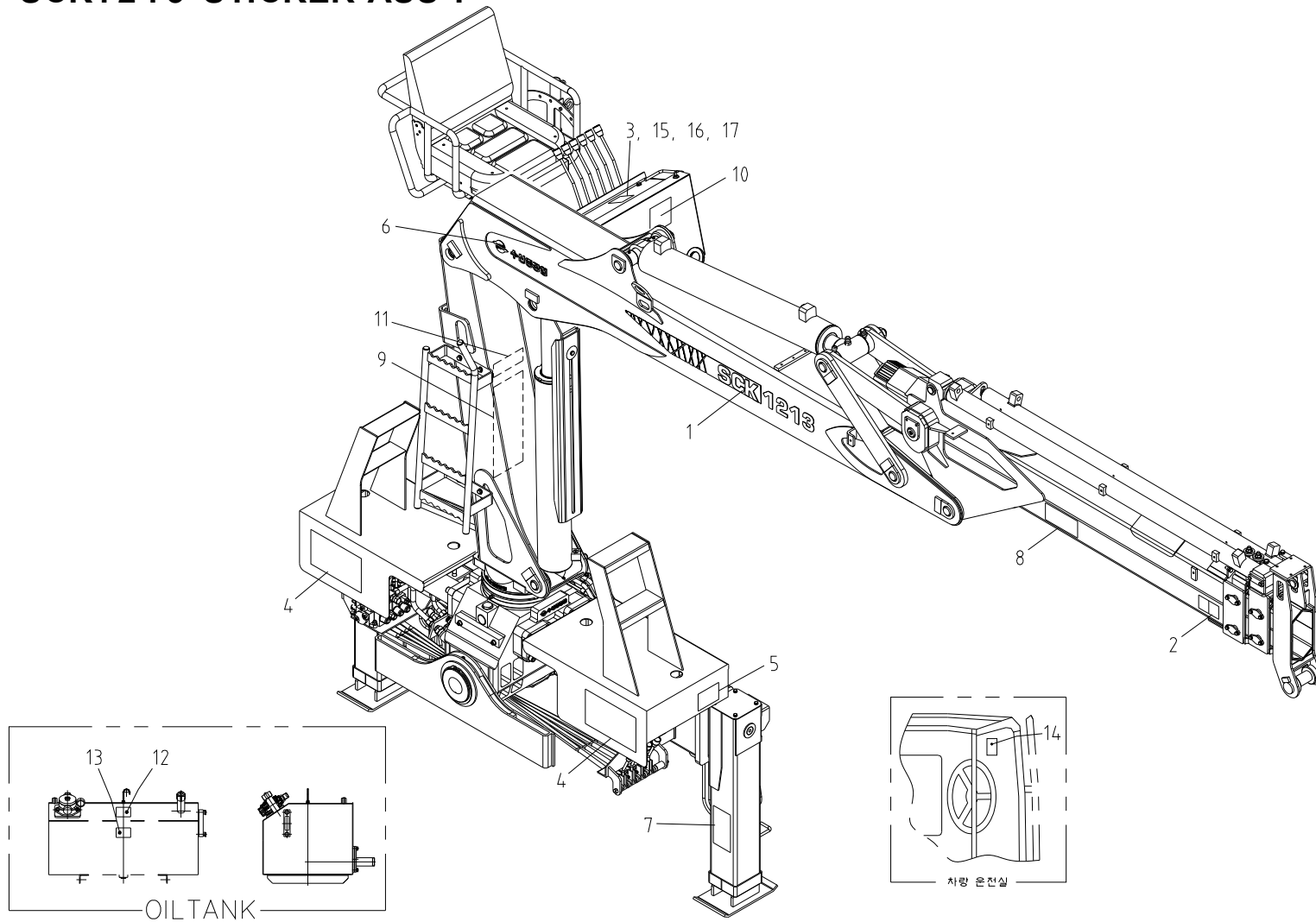
스티커 조립체 Fig. 5 SCK1213 STICKER ASS'Y
