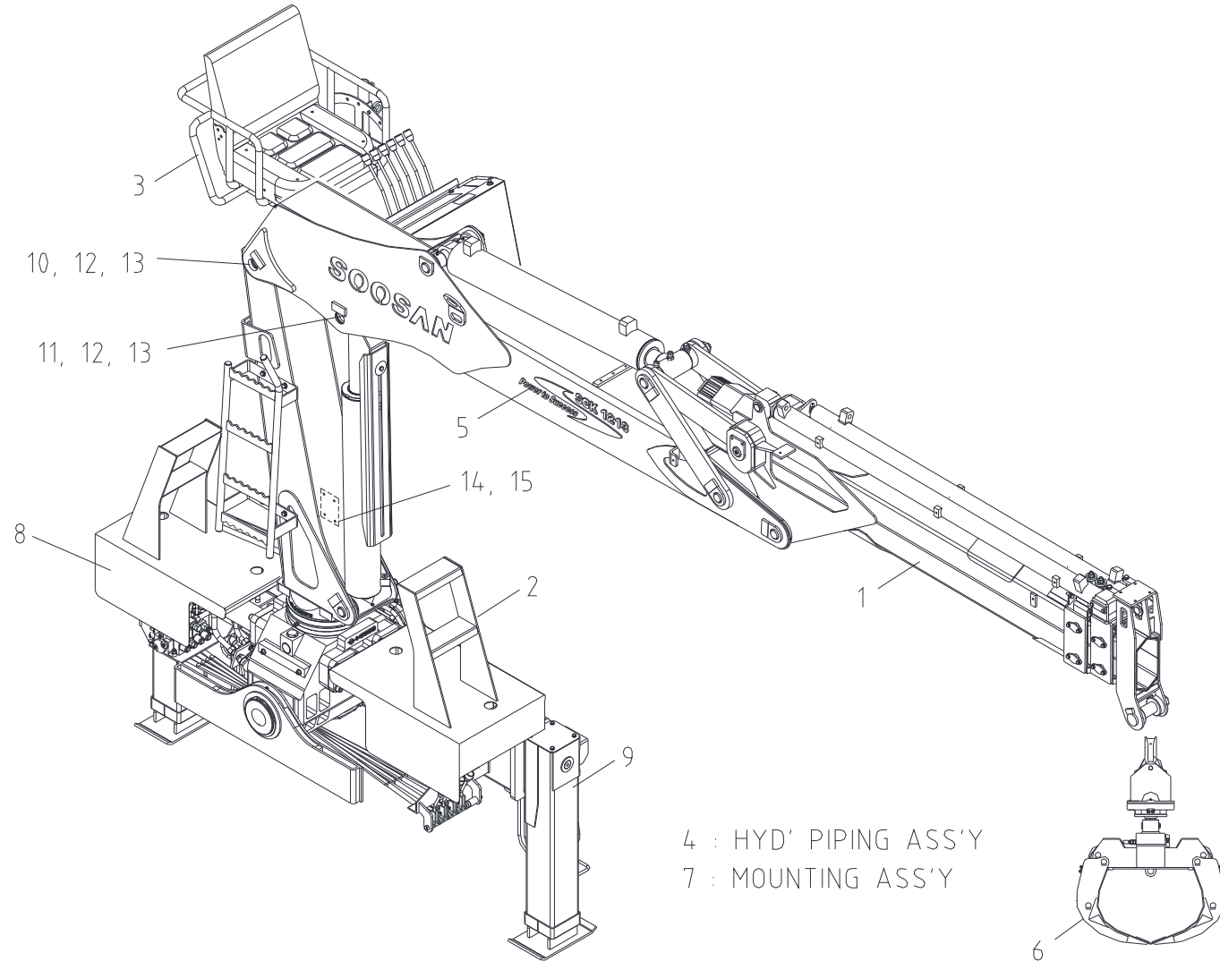
크레인 조립체 Fig. 0 SCK1213 CRANE ASS'Y
