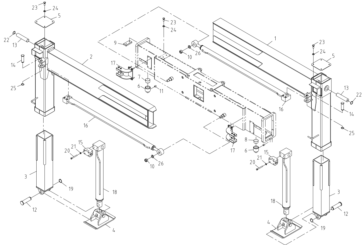
Fig. 9 SCK1213 OUTRIGGER SET
