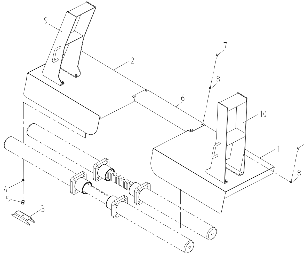
커버 세트 Fig. 8 SCK1213 COVER SET
