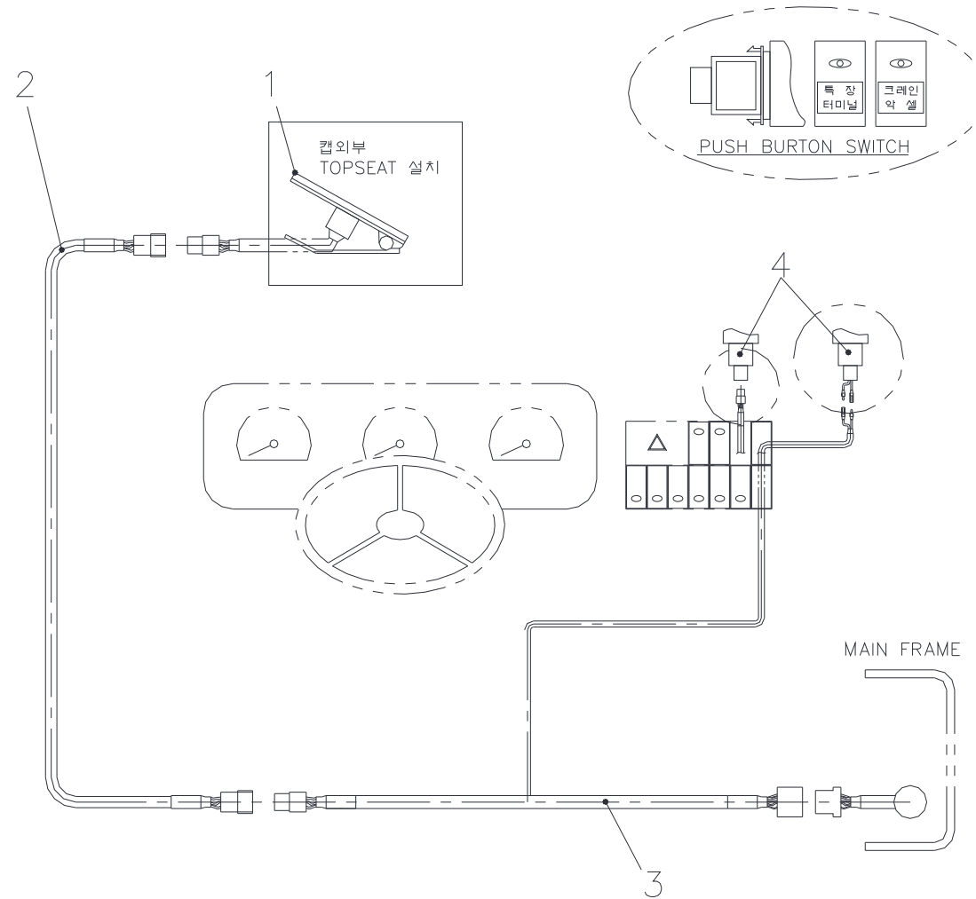
악셀 시스템 셋트 Fig. 7-4 SCK1213 ACC' SYSTEM SET
